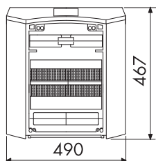
Dimensioni
